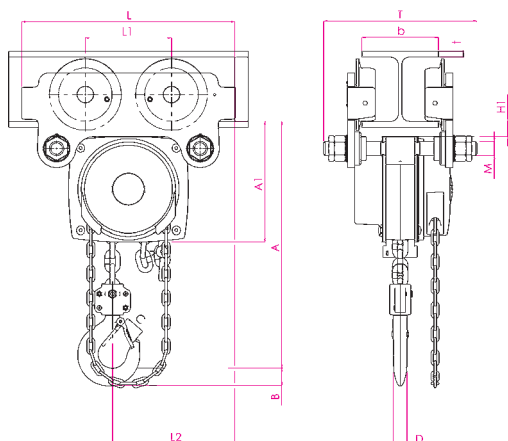
Tip –P, nosivosti 0,5 – 3 t
