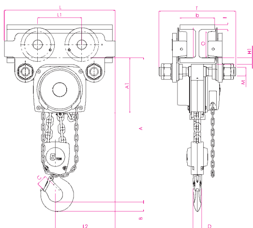
Tip –P, nosivosti 5 t
