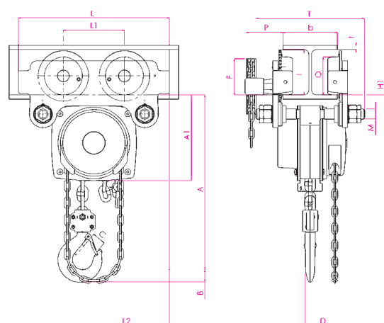
Tip –G, nosivosti 0,5 – 3 t
