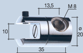
Halter, einseitig drehbar | 1 Shelf holder, single side swivel end Support pivotant 1 face
