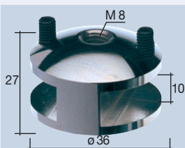
Dekohalter, zweiseitig | 6 Deco holder, double side Support déco 2 faces
